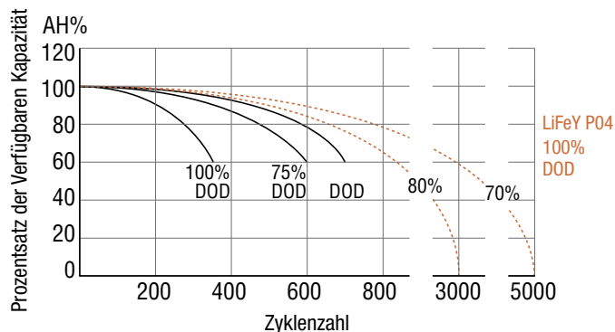
Zyklengebrauchsdauer in Abhängigkeit von der Entladetiefe
