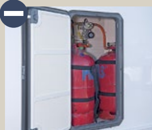
Gasflaschenkasten vorschriftengerecht, aber mit schmaler Tür.
