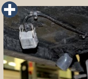
Elektrischer Abwasser-Ablasshahn im Blick der optionalen Kamera.
